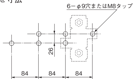
組合せ寸法
