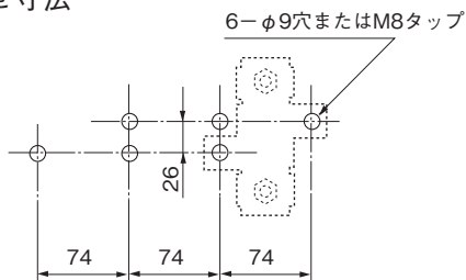
組合せ寸法
