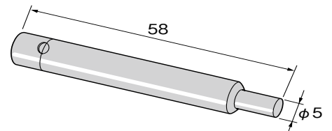
重量 : 3.2g (T-4.2・T-5用)
