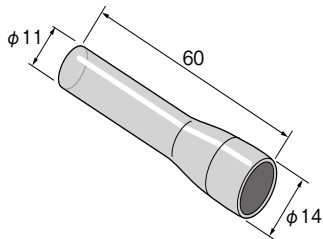
重量 : 8.5g (T-10・T-14用)
