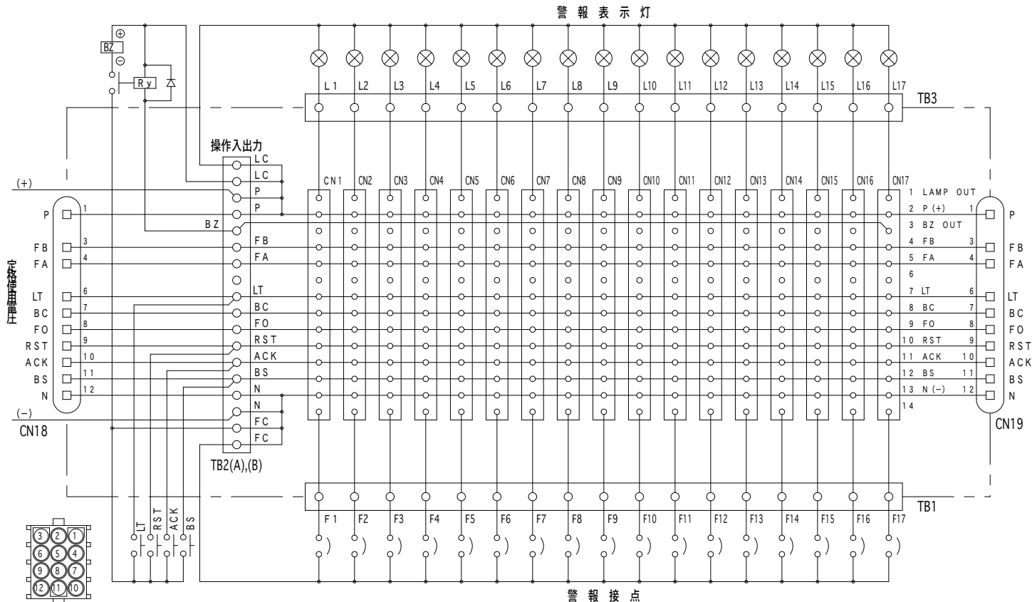
CN18 / CN19 番号図
