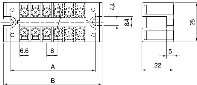
寸法表 (単位:mm)
