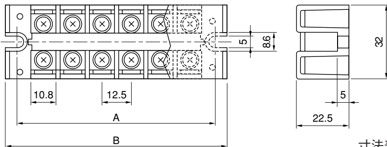
寸法表 (単位:mm)
