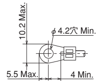
圧着端子寸法
